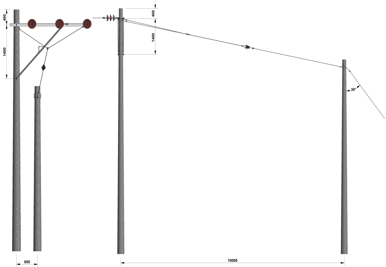
Figura 2. Vista frontal.
