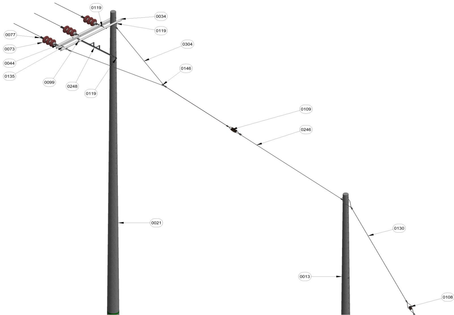
Figura 1. Vista isometrica.
