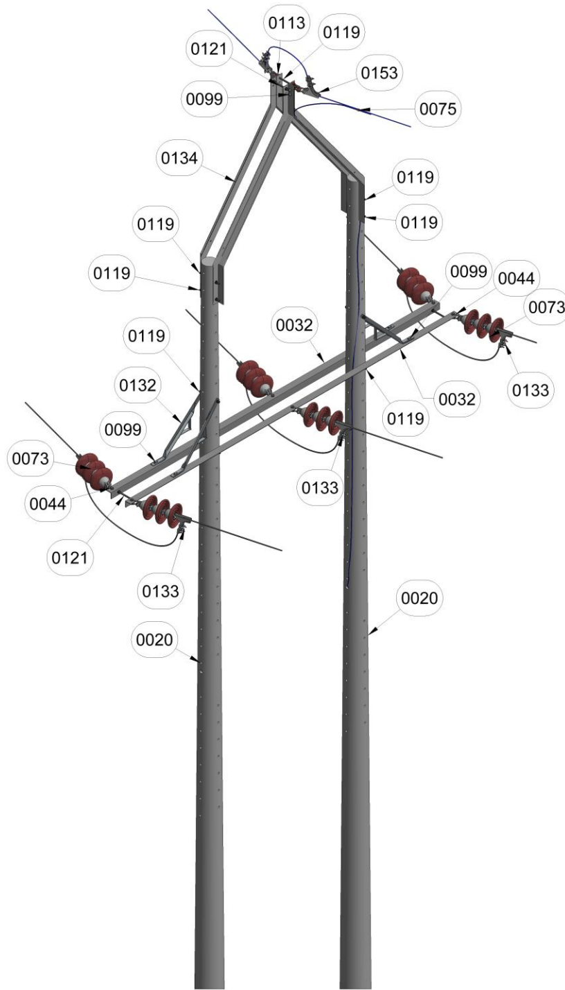
Figura 1. Vista isometrica.
