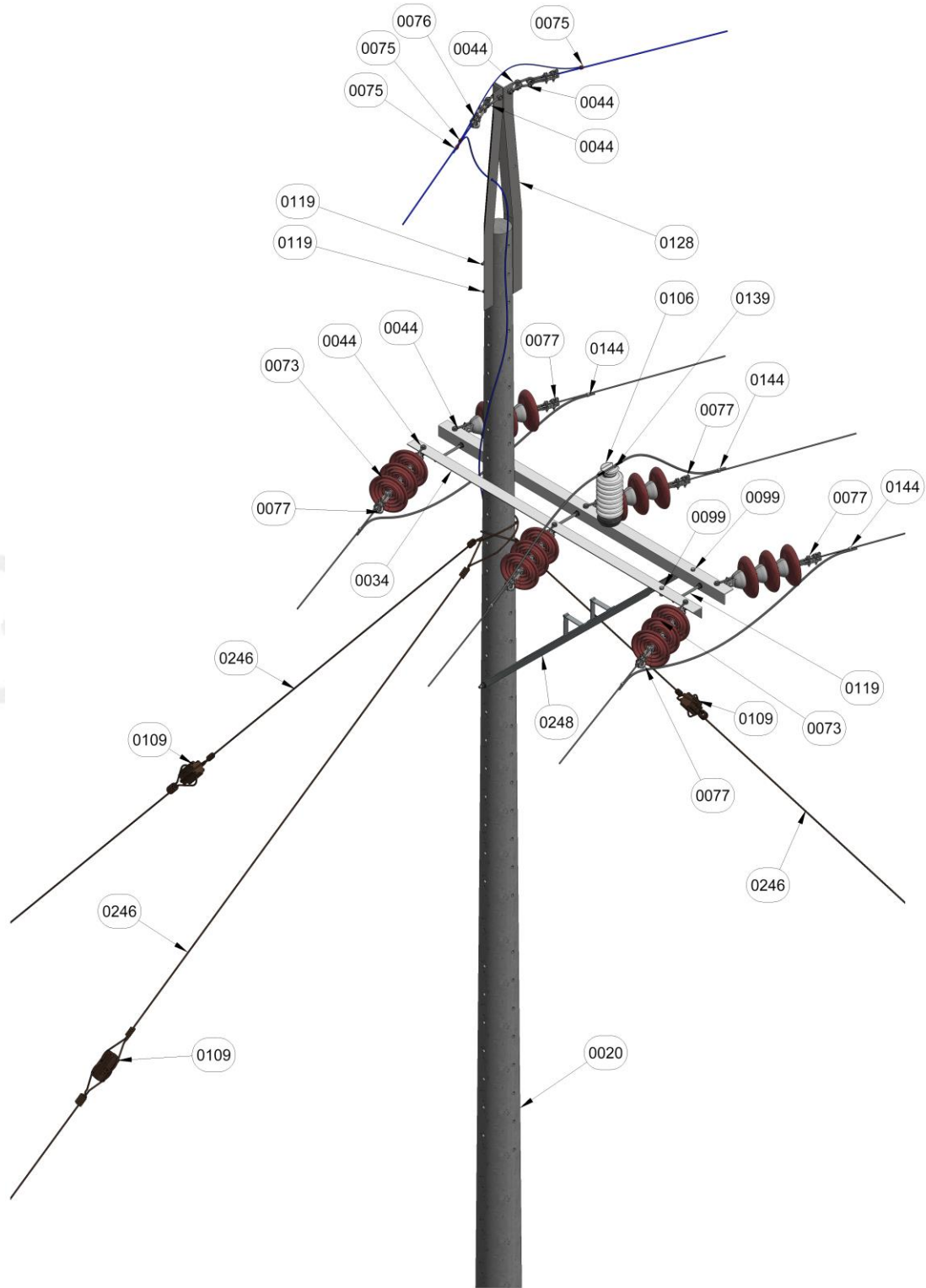
Figura 1. Vista isometrica.
