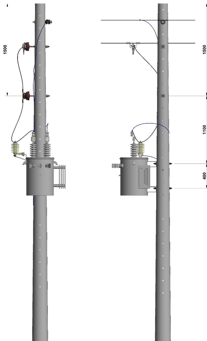
Figura 2. Vista frontal.
