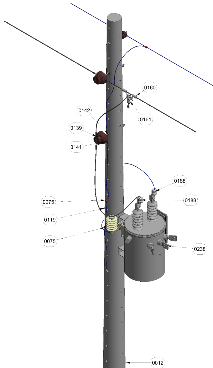
Figura 1. Vista isometrica.
