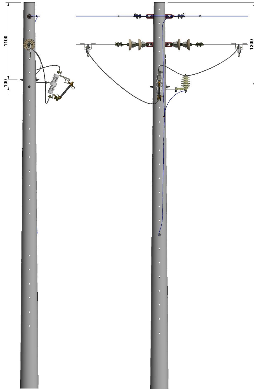
Figura 2. Vista frontal.
