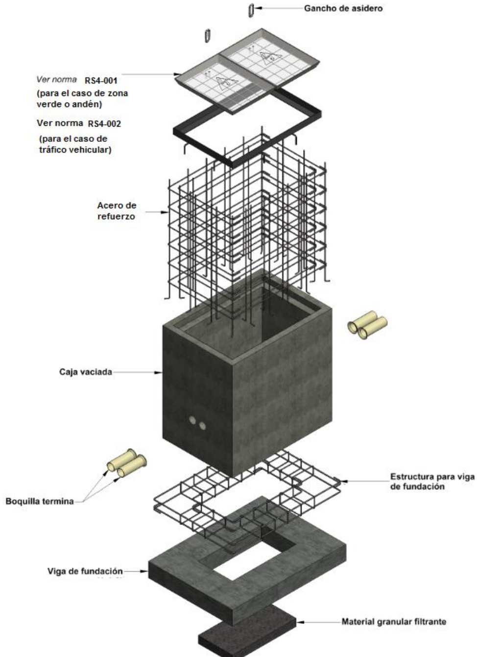
Esquema 2: Cajas vaciadas en concreto – Configuración
