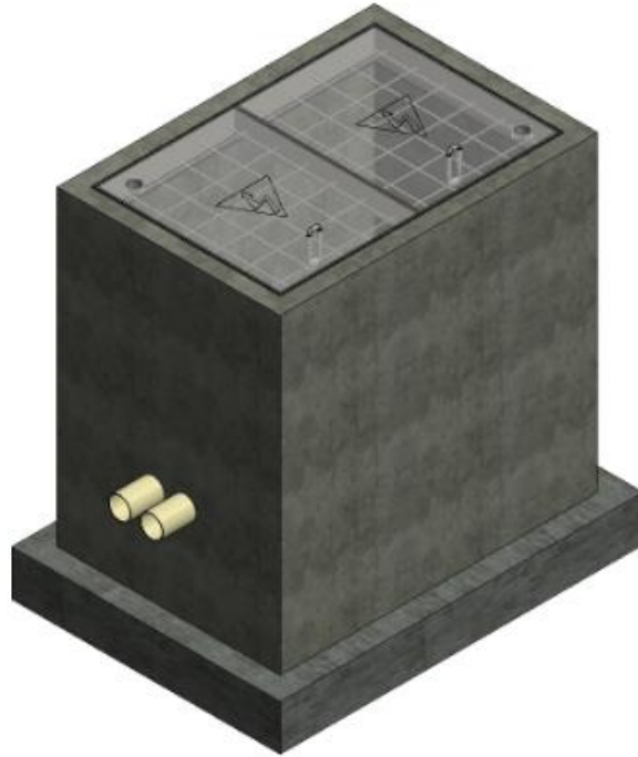
Esquema 1: Cajas vaciadas en concreto – Isométrico
