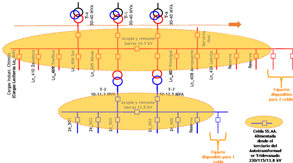
Figura 36. Diagrama unifilar adecuaciones proyecto SE Palenque
