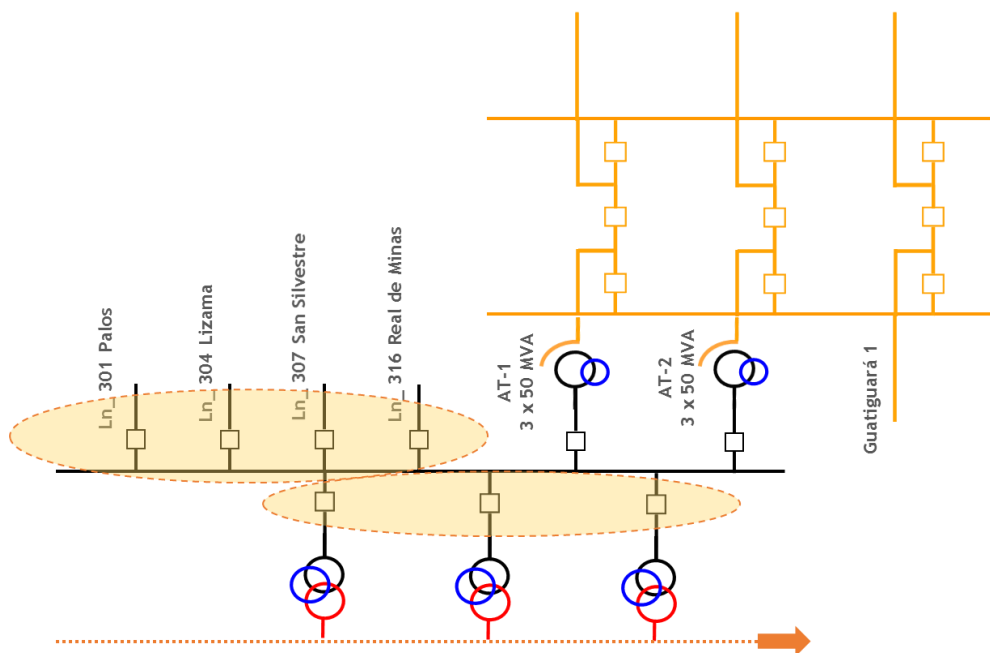
Figura 35. Diagrama unifilar adecuaciones proyecto SE Palenque
