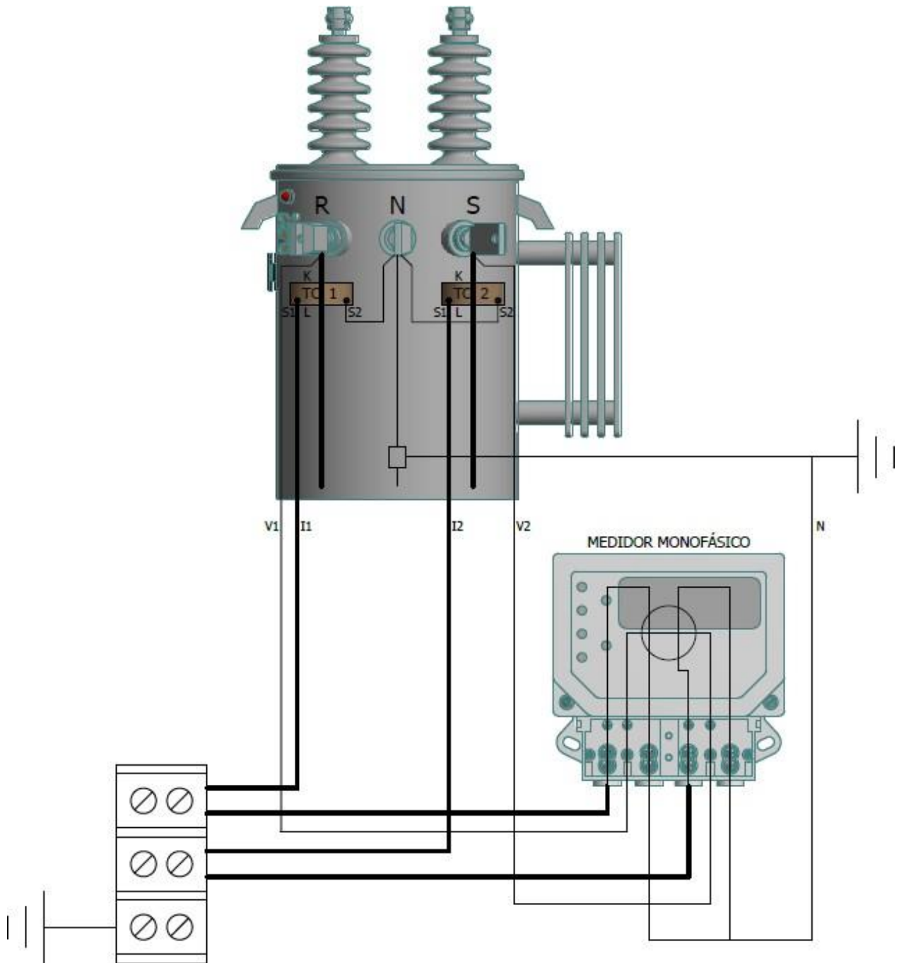
Figura 3. Diagrama de conexión macromedición con medida semi-directa en transformador monofásico medidor de conexión asimétrica o europea. Transformadores existentes, sin TC's internos.
