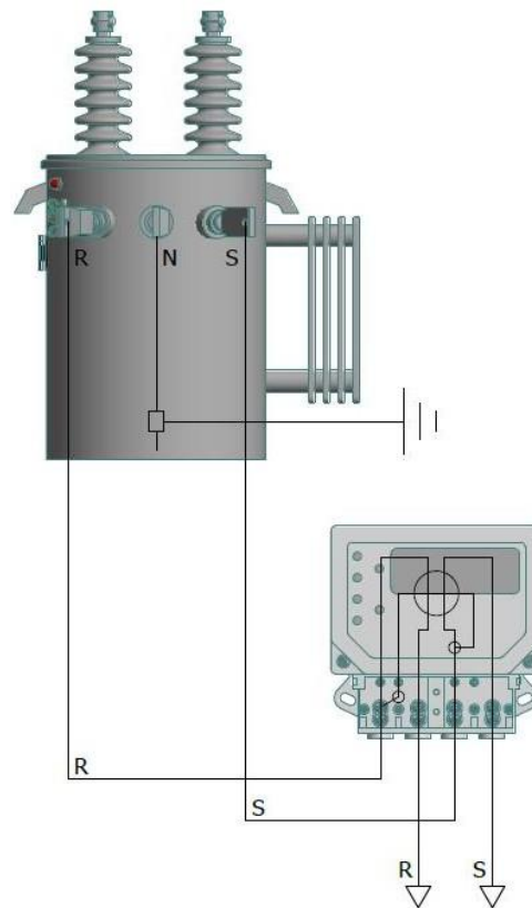
Figura 1. Diagrama de conexión macromedición con medida directa en transformador monofásico potencia menor a 15 kVA, medidor de conexión asimétrica o europeo.
