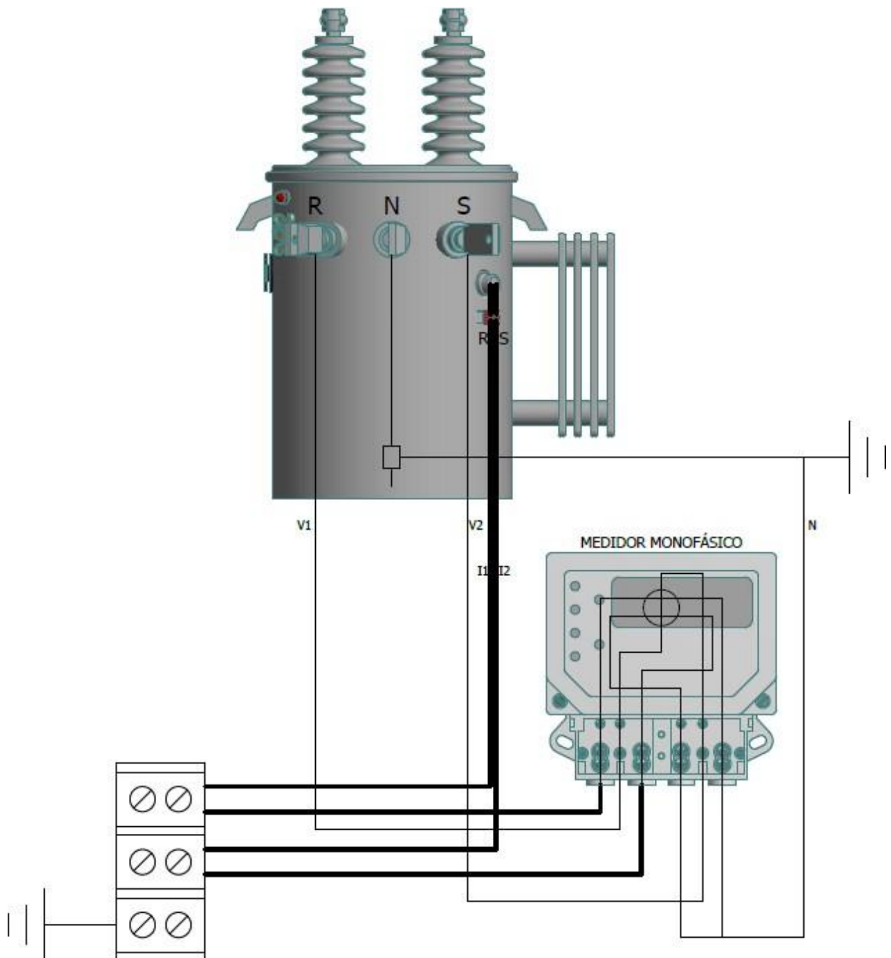
Figura 6. Diagrama de conexión macromedición con medida semi-directa en transformador monofásico con medidor de conexión simétrica o americana. Transformadores nuevos con TC's internos.
