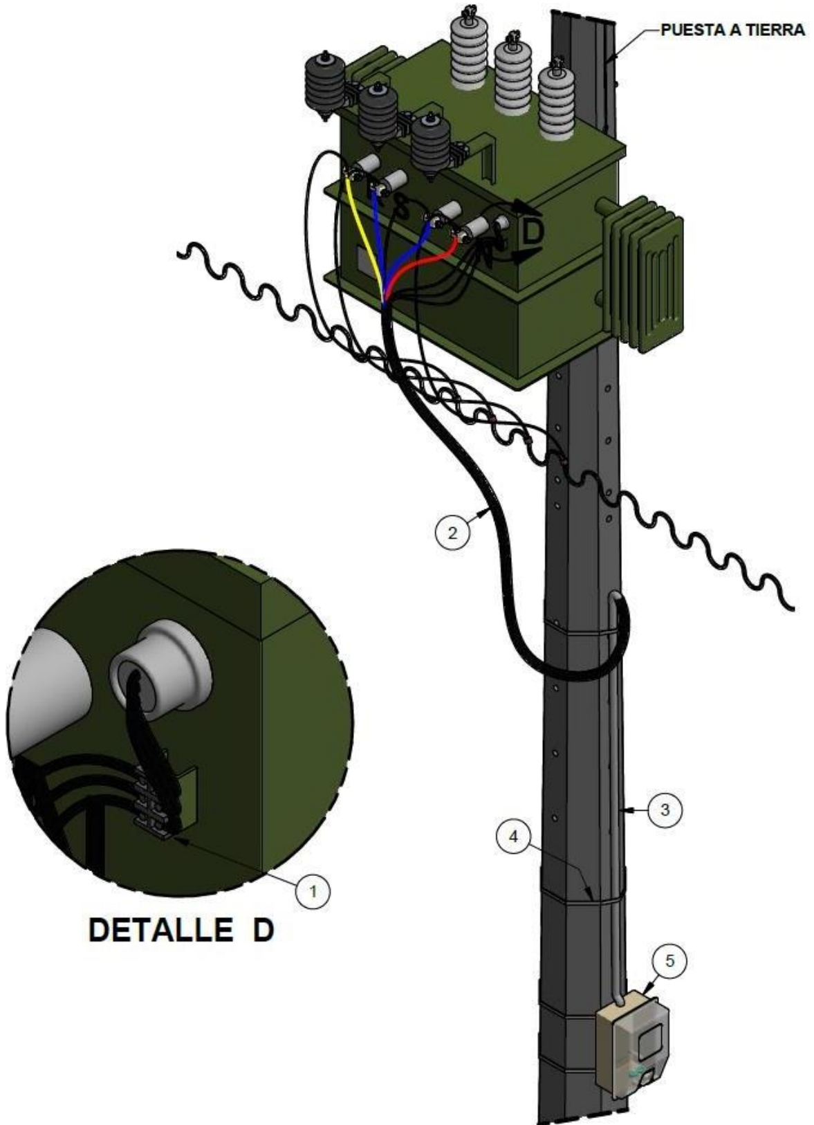
Figura 16. Instalación de macromedidor en transformador trifásico con TC's internos
