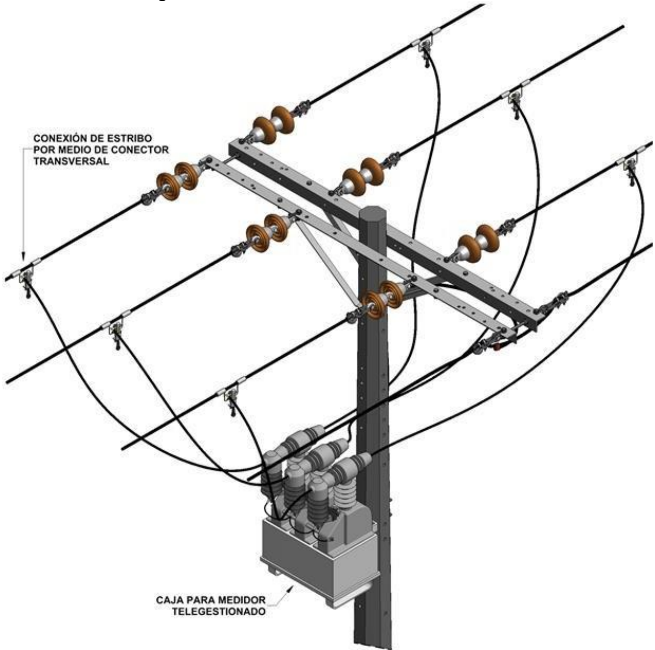
Figura 21. Transformador combinado de medida
