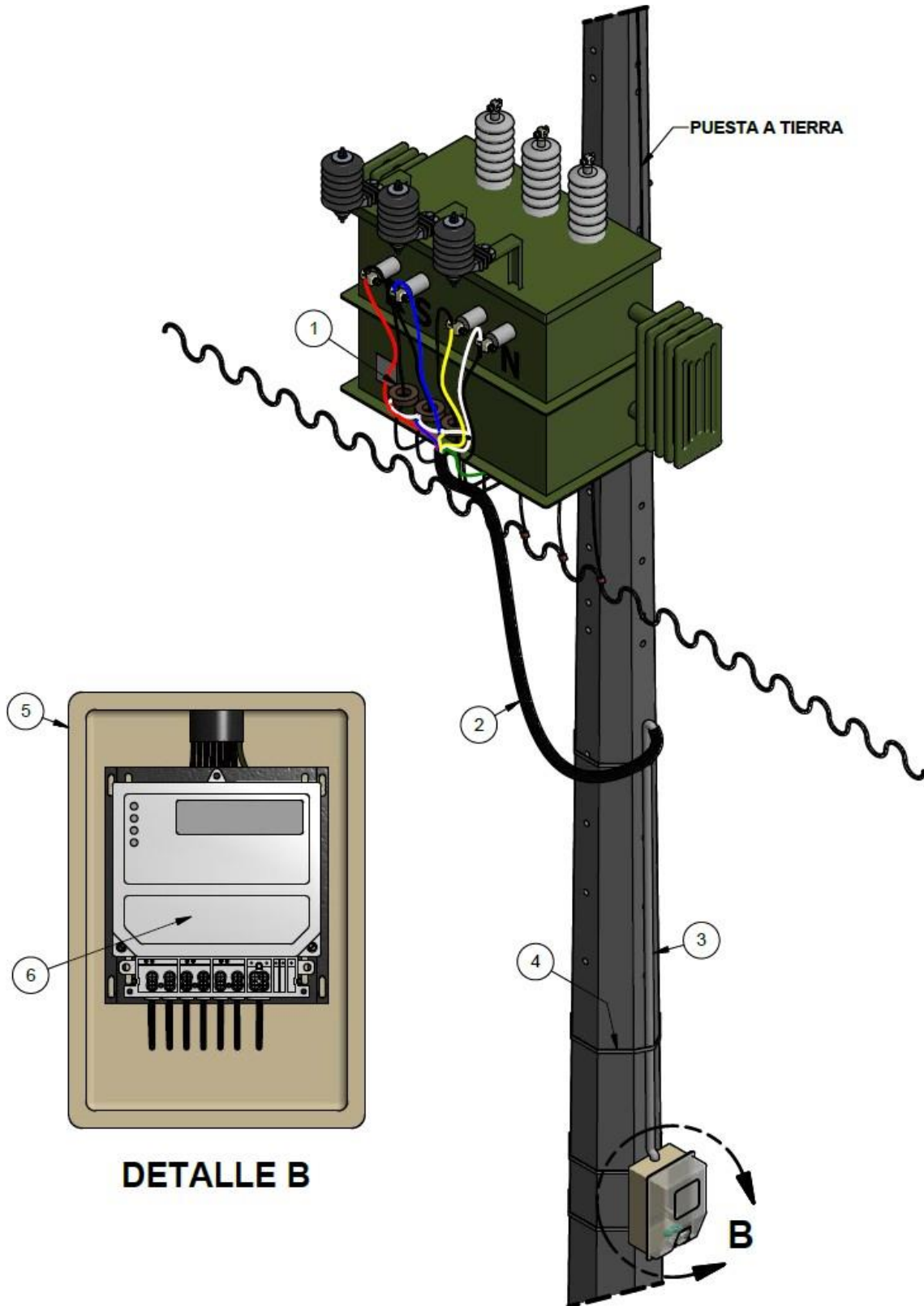
Figura 14. Instalación de macromedidor en transformador trifásico con TC's externos
