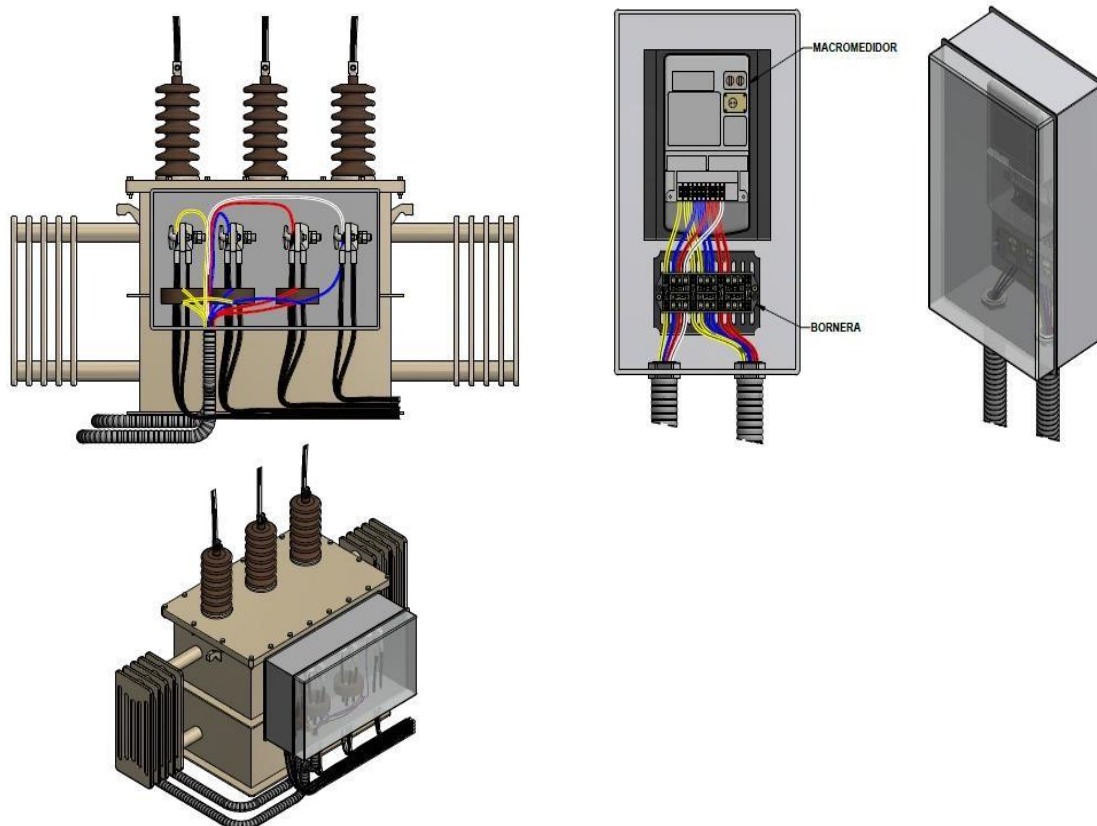
Figura 17. Instalación de macro medición en subestación interna
