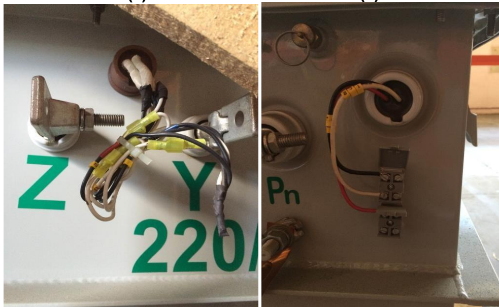
Figura 11. Transformador de distribución con TC's internos, terminales de conexión (1) en cable y (2) con bornera de conexión
