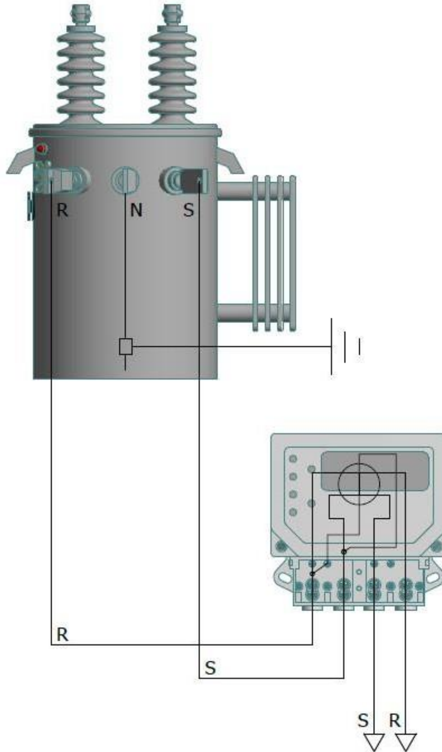
Figura 2. Diagrama de conexión macromedición con medida directa en transformador monofásico potenciamenor a 15 kVA, medidor de conexión simétrica o americana.
