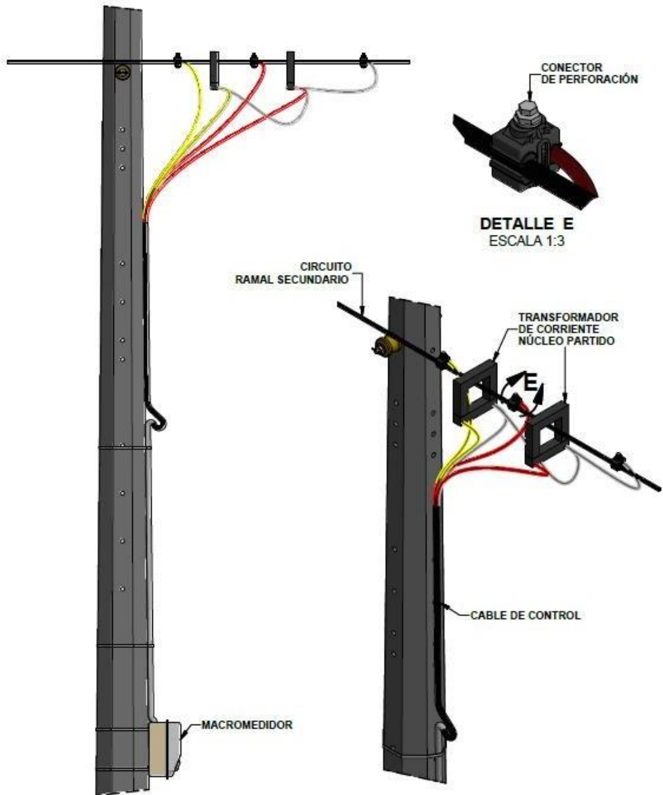
Figura 18. Instalación de macromedición en un circuito ramal
