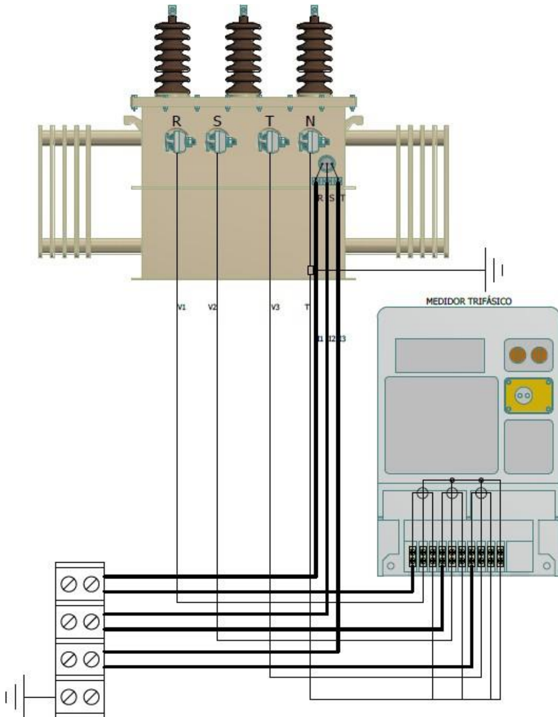
Figura 10. Diagrama de conexión macromedición con medida semi-directa en transformador de distribución trifásico medidor de conexión simétrica o americana. Transformadores nuevos con TC's internos.
