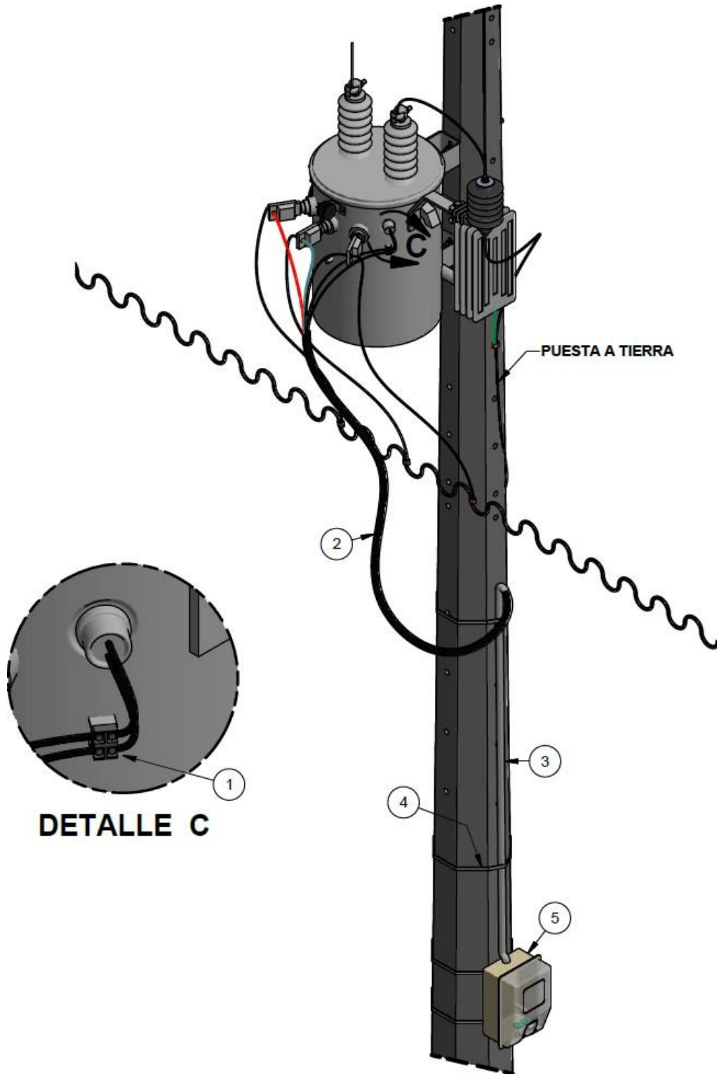
Figura 15. Instalación de macromedidor en transformador monofásico con TC's internos
