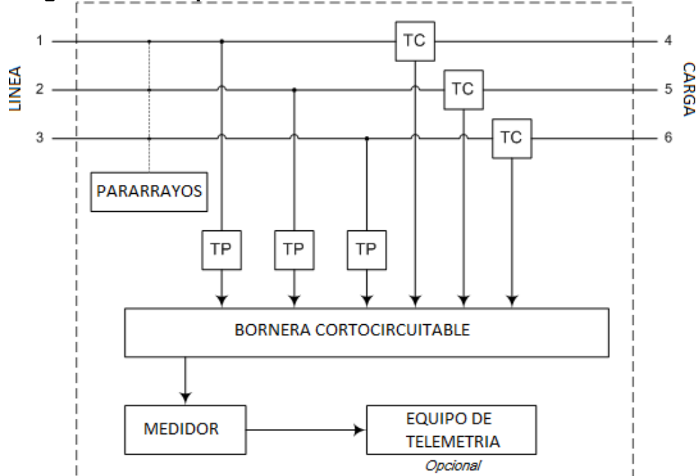
Figura 20. Principio de funcionamiento del sistema combinado
