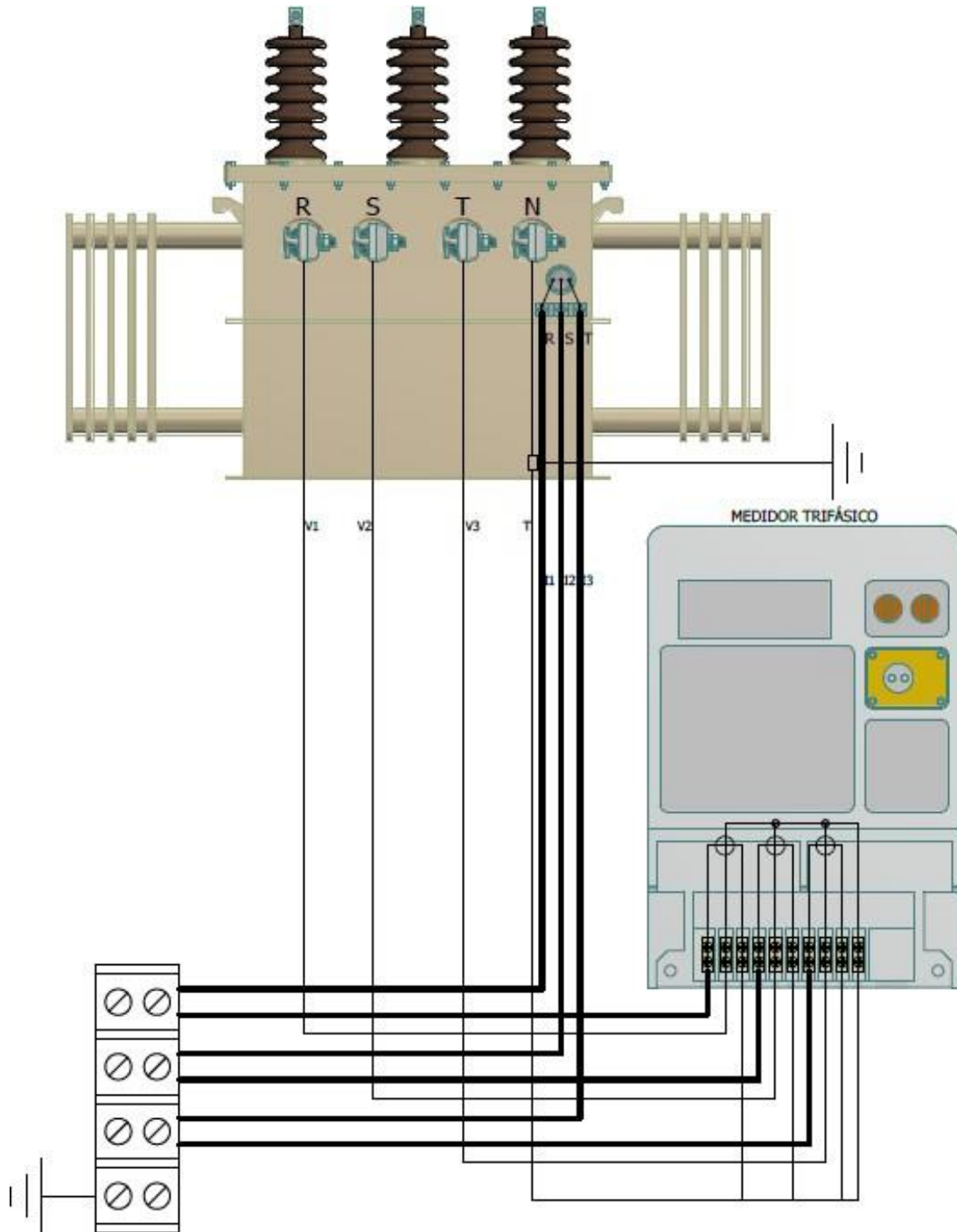
Figura 8. Diagrama de conexión macromedición con medida semi-directa en transformador de distribución trifásico, medidor de conexión asimétrica o europea. Transformadores nuevos con TC's internos.
