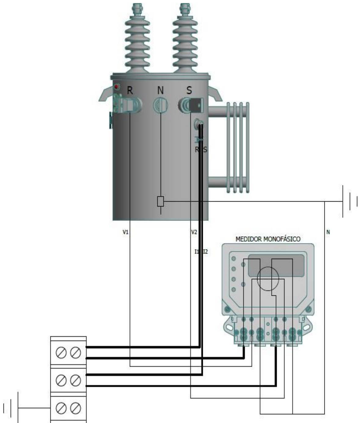
Figura 4. Diagrama de conexión macromedición con medida semi-directa en transformador monofásico con medidor de conexión asimétrica o europea. Transformadores nuevos con TC's internos.
