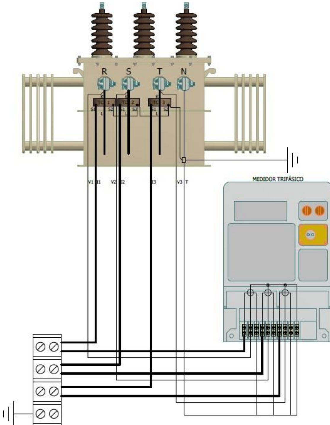
Figura 7. Diagrama de conexión macromedición con medida semi-directa en transformador de distribución trifásico medidor de conexión asimétrica o europea. Transformadores existentes sin TC's internos.
