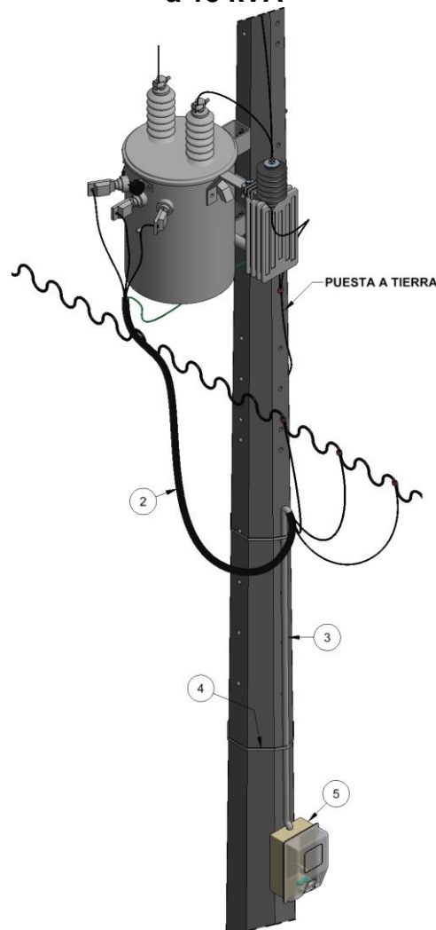
Figura 12. Instalación de macromedidor en transformador 1F con potencia menor o igual a 15 kVA
