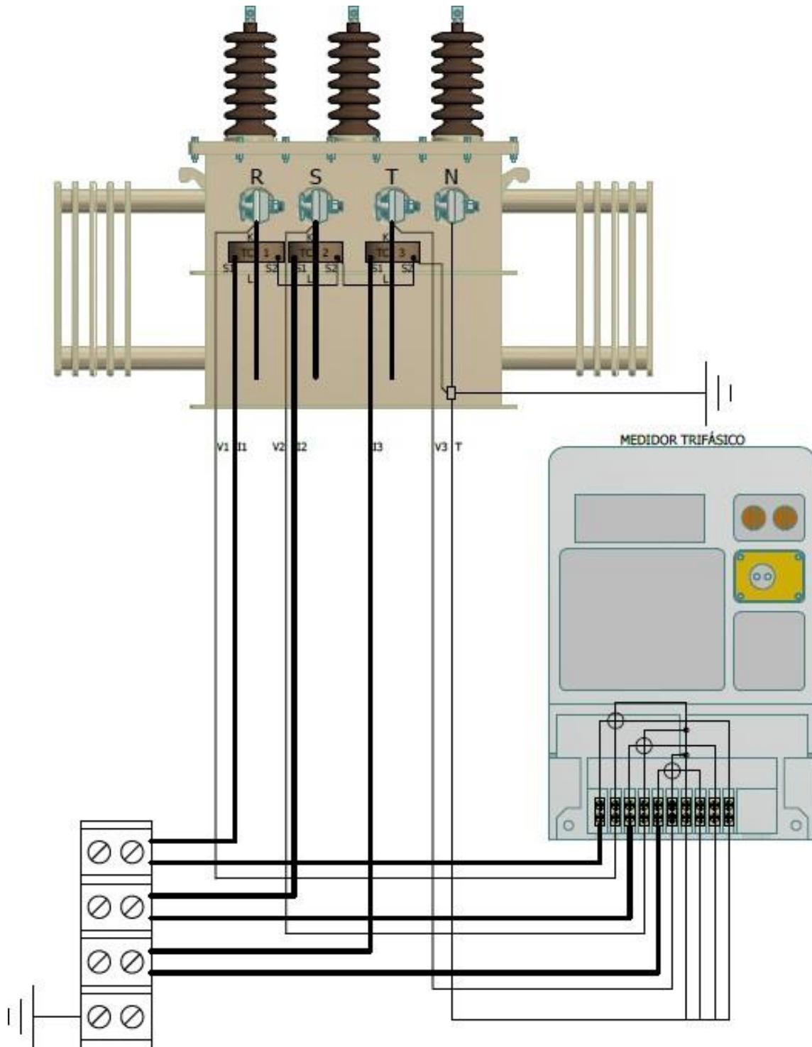
Figura 9. Diagrama de conexión macromedición con medida semi-directa en transformador de distribución trifásico medidor de conexión simétrica o americana. Transformadores existentes sin TC's internos.
