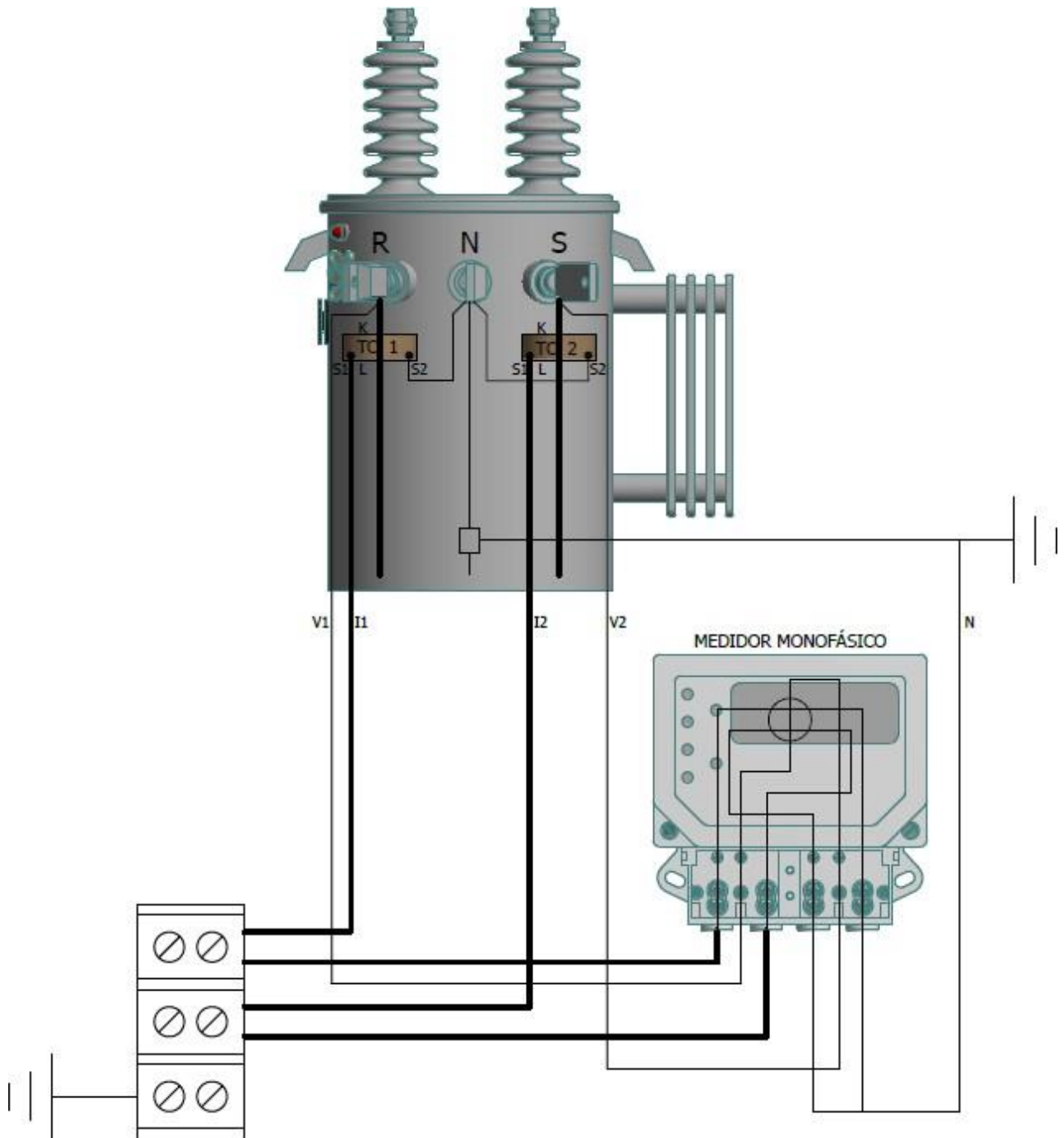
Figura 5. Diagrama de conexión macromedición con medida semi-directa en transformador monofásico medidor de conexión simétrica o americana. Transformadores existentes, sin TC's internos.
