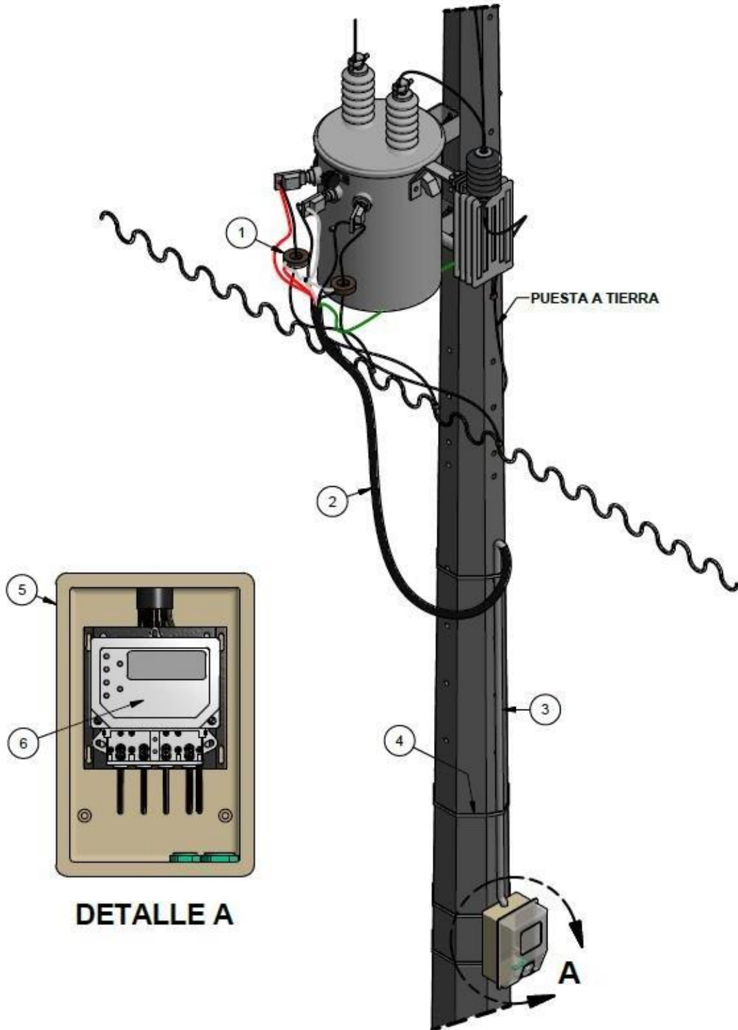
Figura 13. Instalación de macromedidor en transformador monofásico con TC's externos
