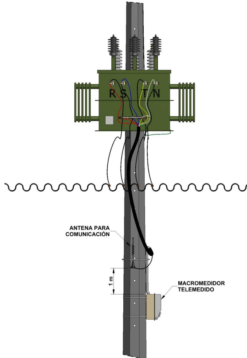
Figura 19. Instalación de medidor integrador telemedido en transformador trifásico con TC's externos
