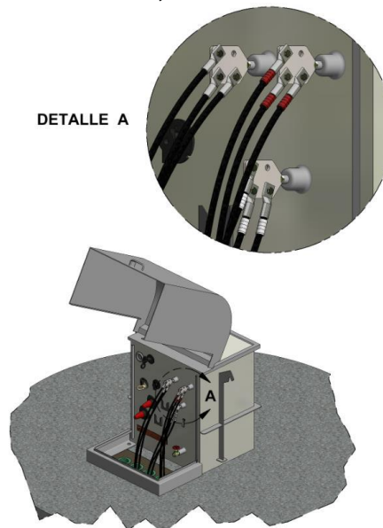
Figura 8. Transformador Pad Mounted, alimentación red secundaria subterránea
