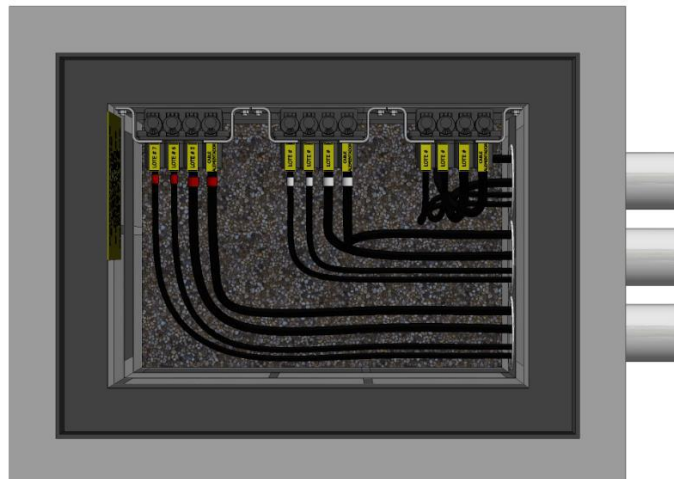
Figura 6. Instalación barrajes secundarios de derivación (3x4) en caja
