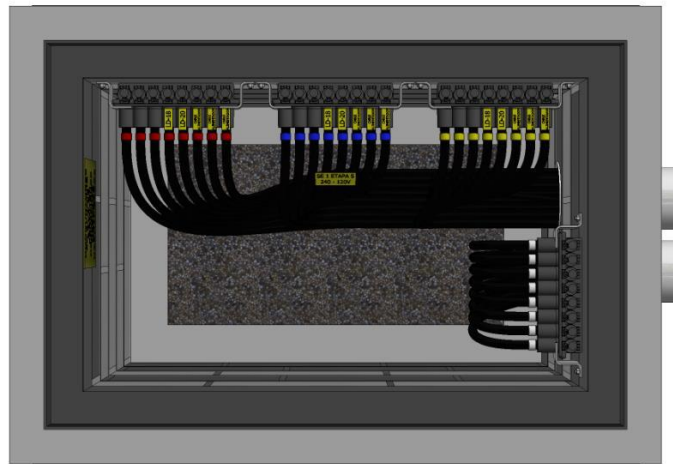
Figura 7. Instalación de barrajes secundarios de derivación (4x8) en caja
