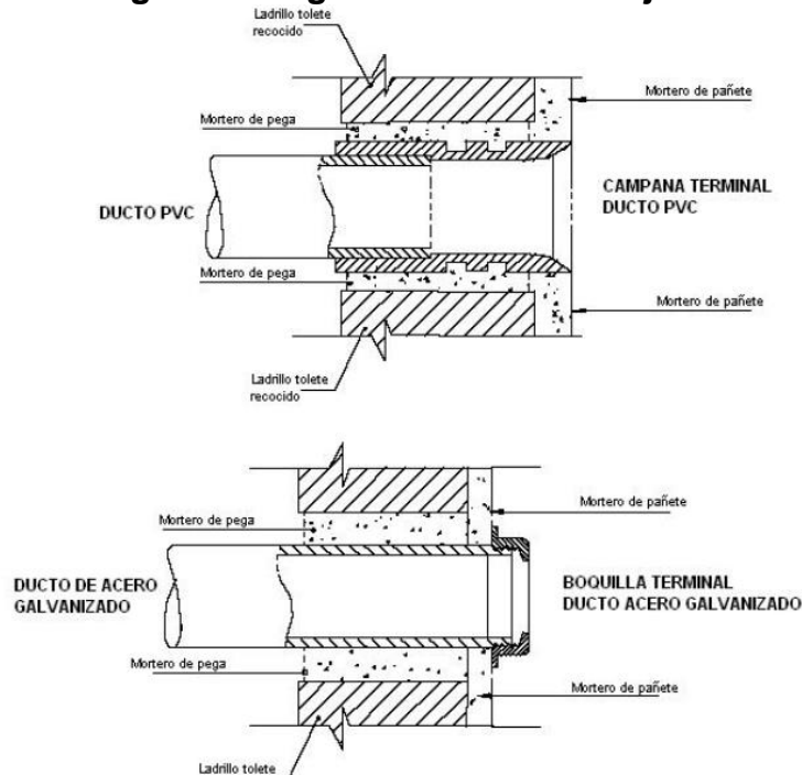
Figura 9. Llegada de ductos a cajas
