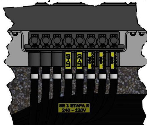
Figura 4. Barraje de derivaciones de 8 vías
