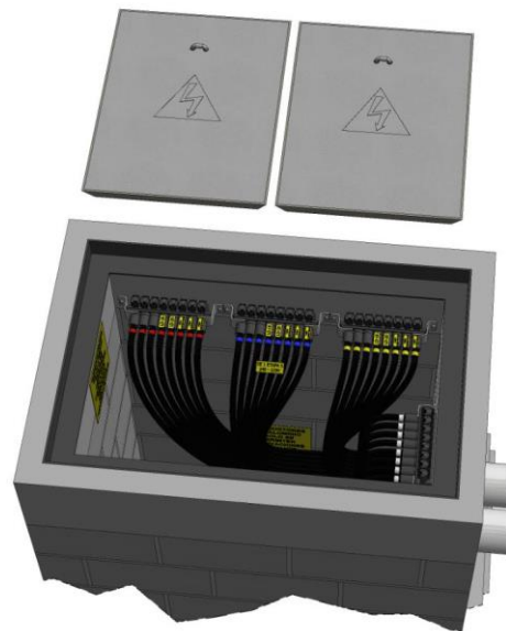
Figura 3. Caja y barraje de derivaciones
