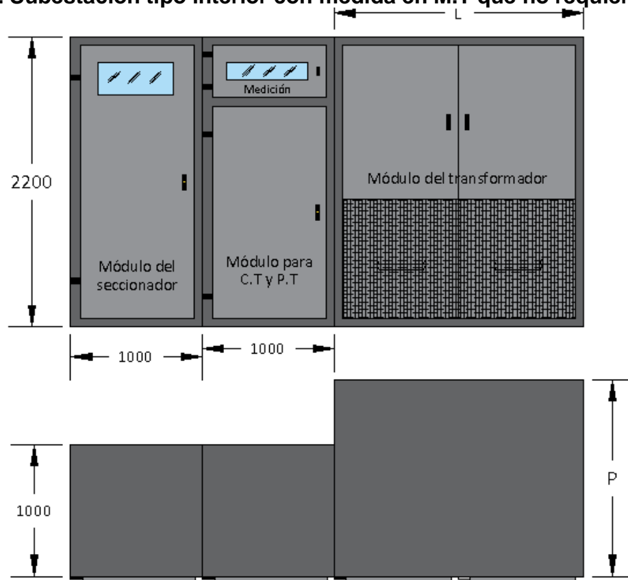
Figura 8. Subestación tipo interior con medida en M.T que no requiere bóveda.
