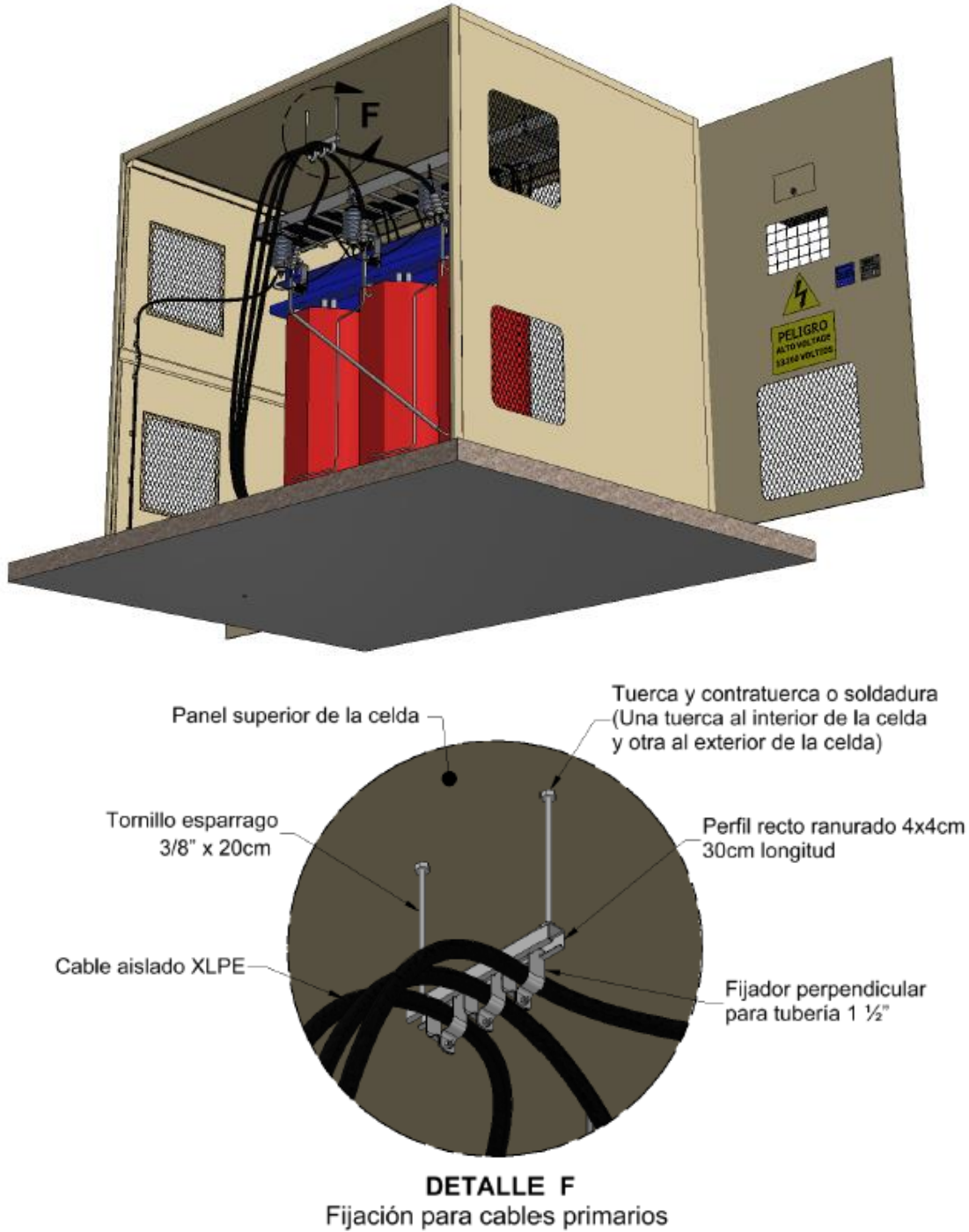
Figura 1. Soporte de sujeción para los conductores de media tensión.
