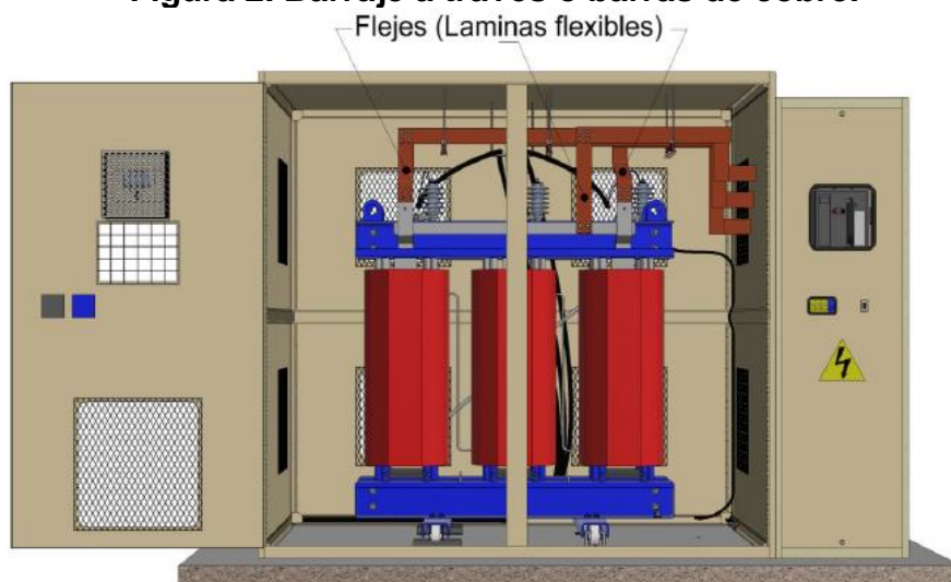
Figura 2. Barraje a través o barras de cobre.
