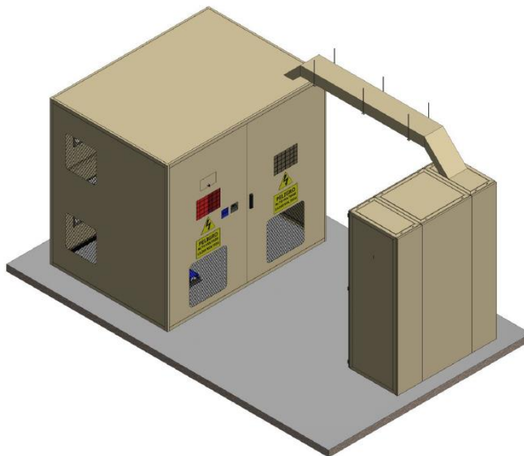
Figura 4. Instalación de celda del transformador en frente al tablero principal.
