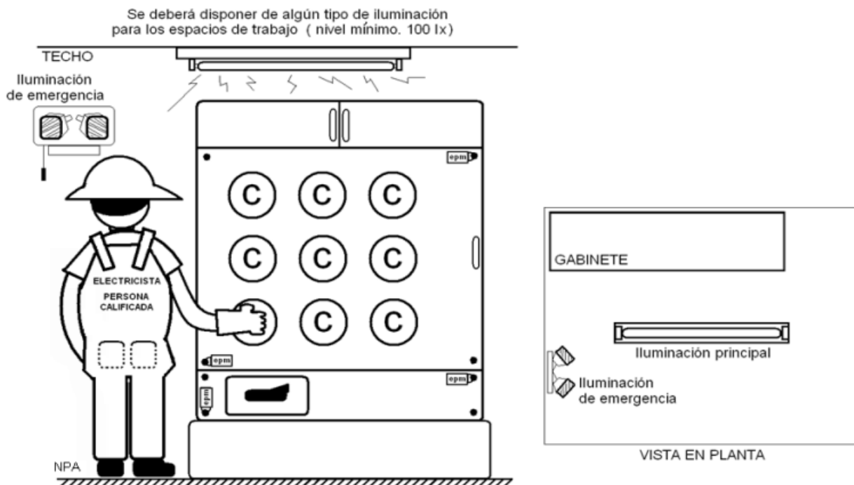
Figura 6. Iluminación para subestaciones tipo interior.
