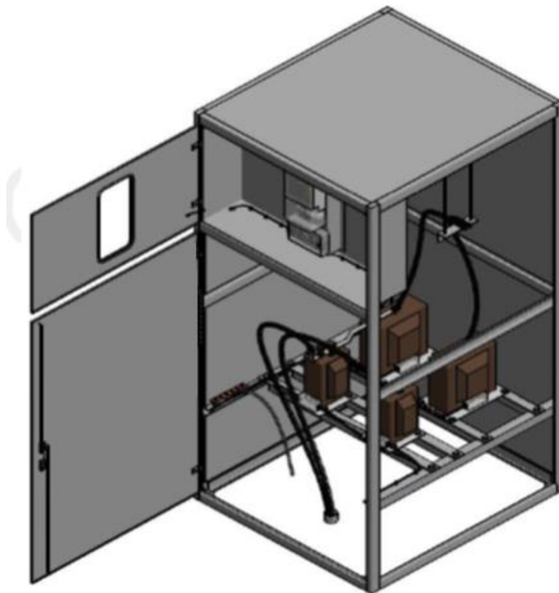
Figura 5. Celda de media tensión de dos (2) elementos.
